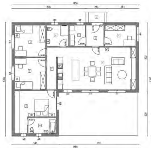
MK TIP 145 BRUTO: 145.88 M2
