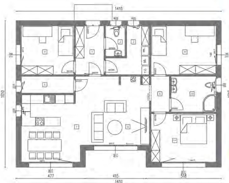
MK TIP 141 BRUTO: 114.39 M2
