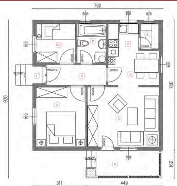
MK TIP 59 BRUTO: 65.59 M2
