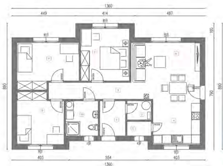
MK TIP 107 BRUTO: 107.48 M2
