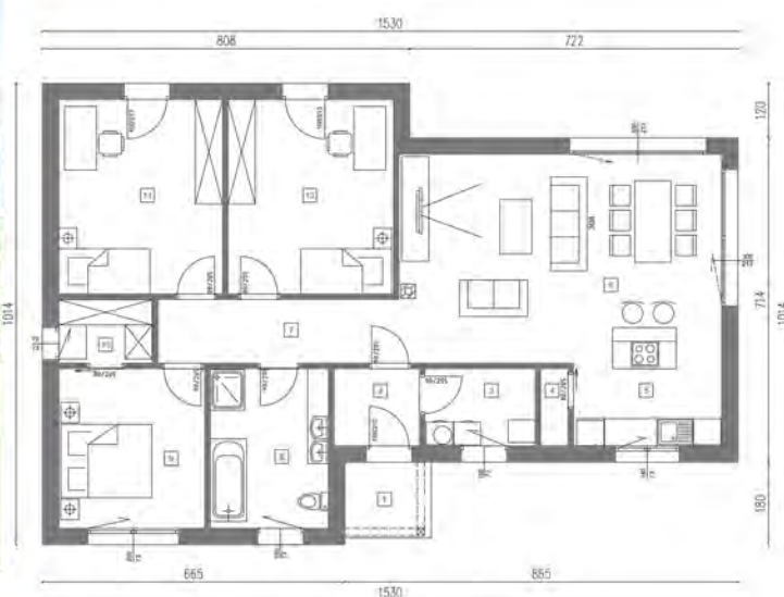
MK TIP 136 BRUTO: 135.28 M2
