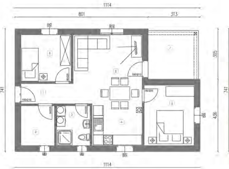
MK TIP 82 BRUTO: 81.99 M2
