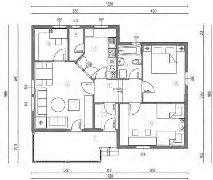
MK TIP 81 BRUTO: 98.05 M2
