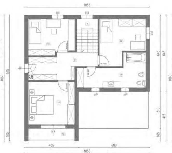
OSNOVA SPRATA MK 187S
