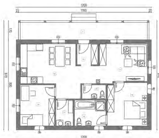
MK TIP 114 BRUTO: 121.44 M2
