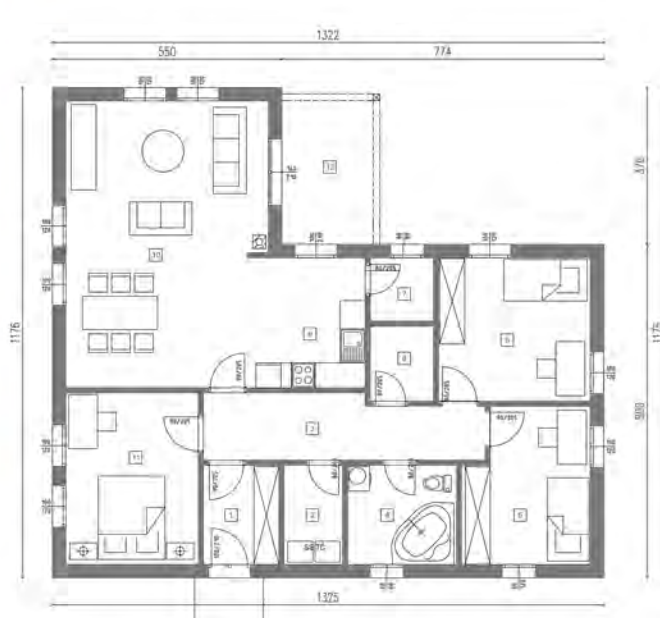
MK TIP 136 BRUTO: 135.28 M2
