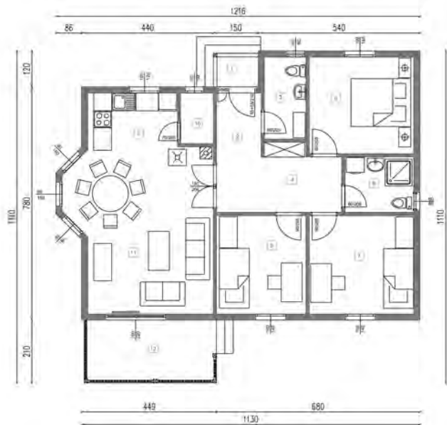
MK TIP 107 BRUTO: 107.48 M2
