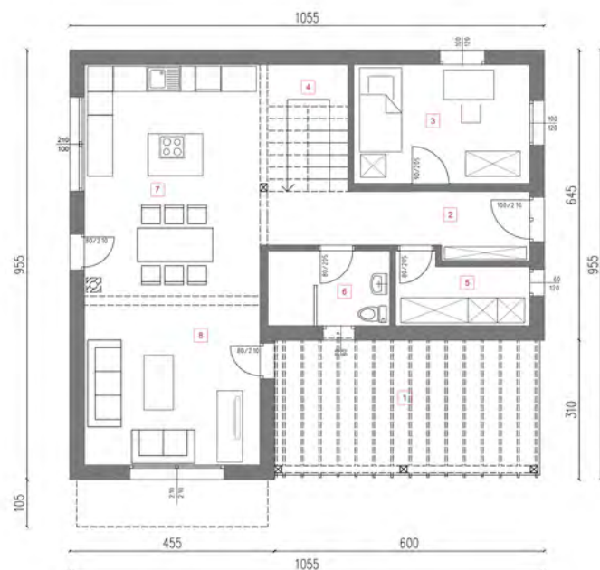
OSNOVA PRIZEMLJA MK 187S
