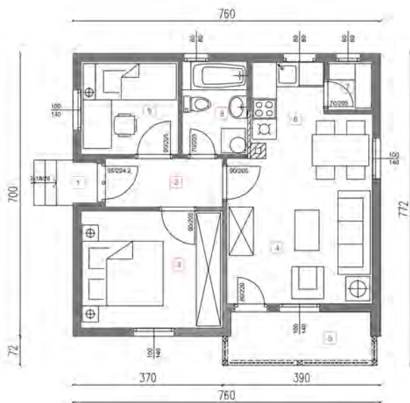
MK TIP 52 BRUTO: 57.05 M2
