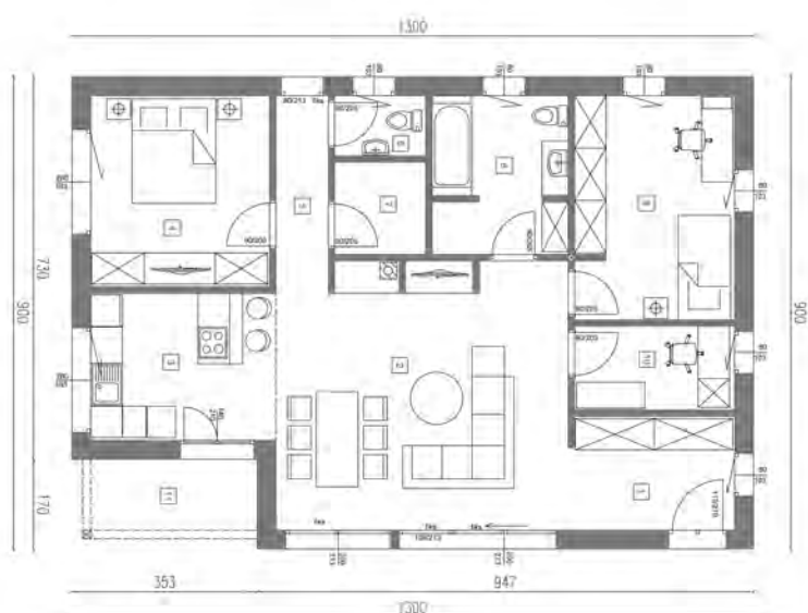
MK TIP 118 BRUTO: 128.45 M2
