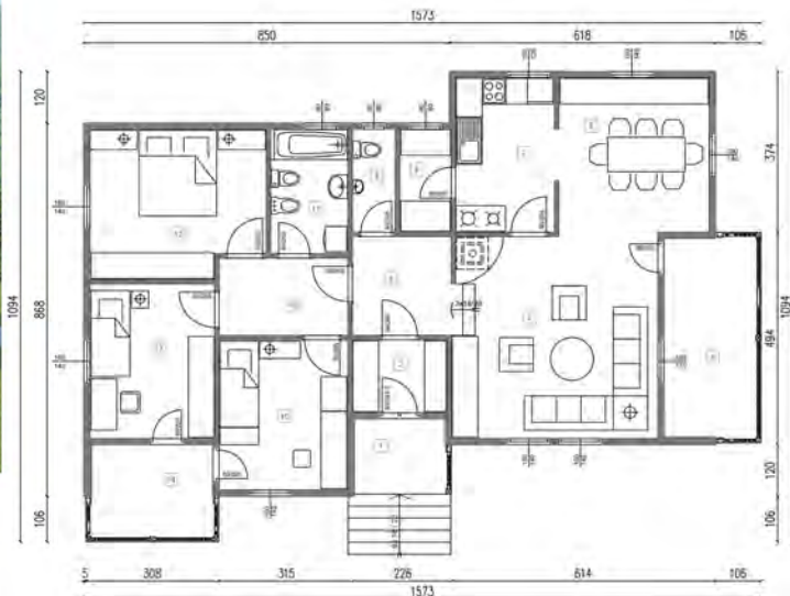
MK TIP 127 BRUTO: 139.16 M2
