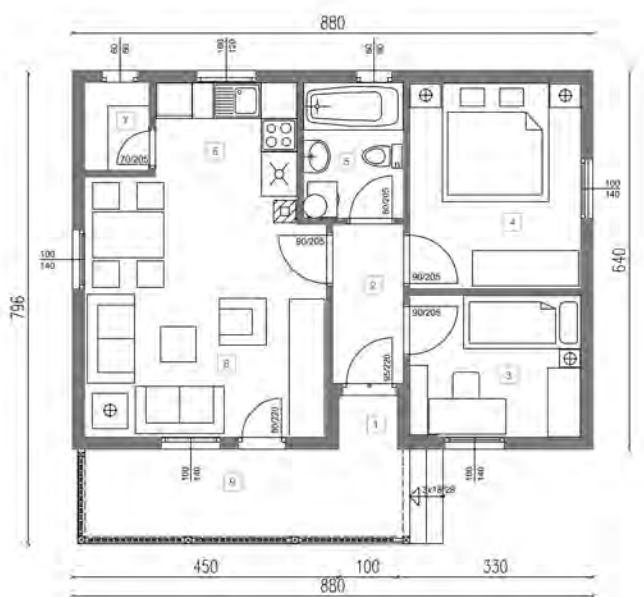
MK TIP 52 BRUTO: 57.05 M2
